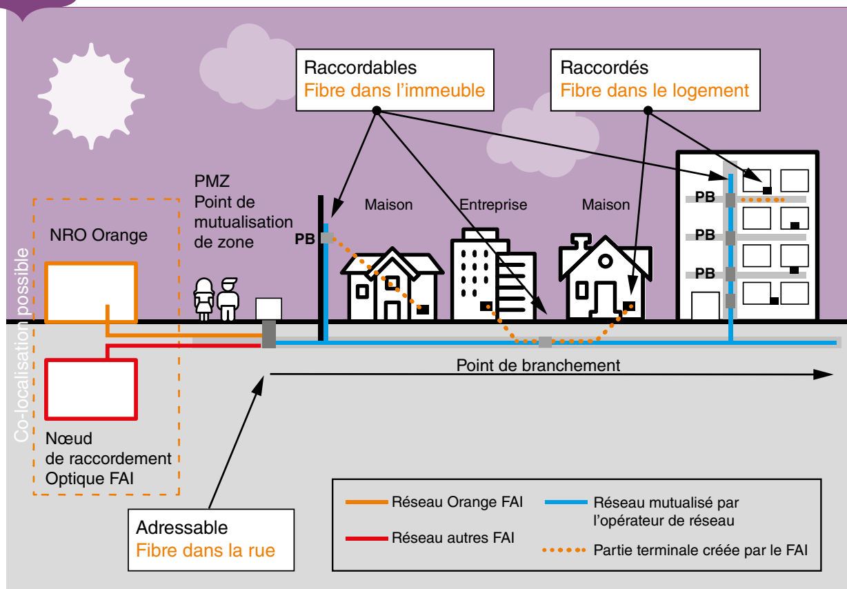
Schéma qui retrace les étapes du déploiement dans la commune
